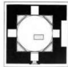
پلان آرامگاه امير ارسلان جاذب
