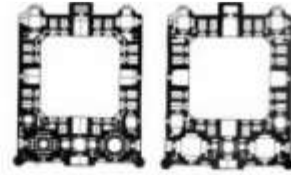
پلان مدرسه غیاثیه خرگرد
