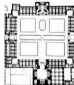
پلان مدرسه چهارباغ
