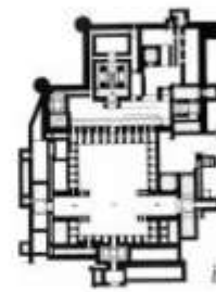
پلان مجموعه کاخ کوه خواجه، سیستان
