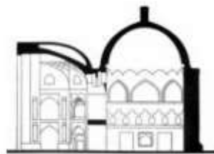
مقطع مسجد جامع قزوین
