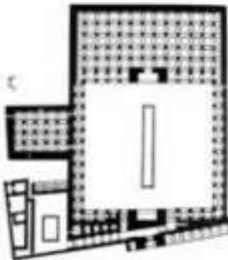
پلان مسجد وکیل شیراز
