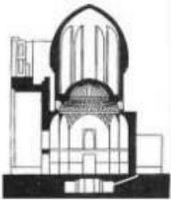
گنبد دو پوسته گسسته
