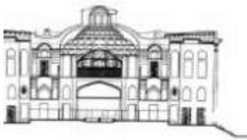
مقطع کاخ هشت‌بهشت
