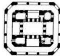
پلان کاخ چهلستون، قزوین
